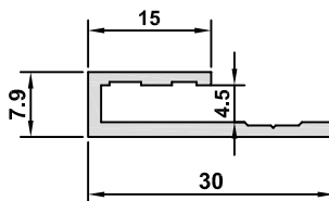
4995-1.6 AĞIRLIK / WEIGHT 0,217 kg/m
