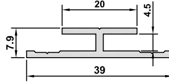
6869-18 AĞIRLIK / WEIGHT 0,284 kg/m
