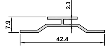
5259-12 AĞIRLIK / WEIGHT 0,205 kg/m
