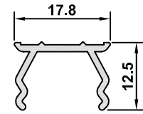
2198-15 AĞIRLIK / WEIGHT 0,140 kg/m
