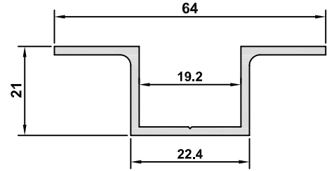
4481-20 AĞIRLIK / WEIGHT 0,561 kg/m
