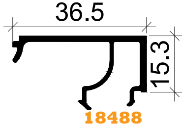
CAM ÇİTALARI GLAZING BEADS
