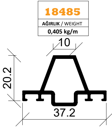
CAM ÇİTALARI GLAZING BEADS
