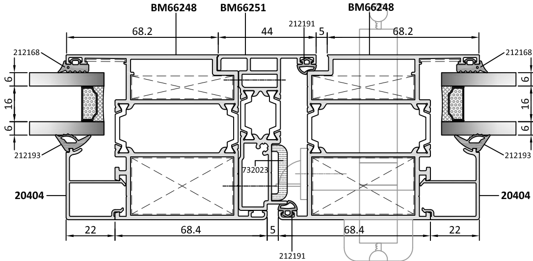
İÇE AÇILIR KAPI INWARD OPENING DOOR
