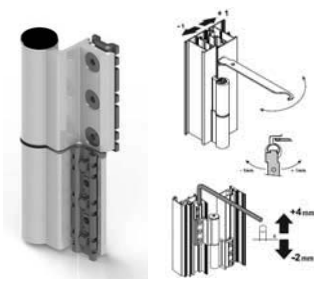
AYARLI KAPI MENTEŞESİ (100 KG) ADJUSTABLE DOOR HINGE
