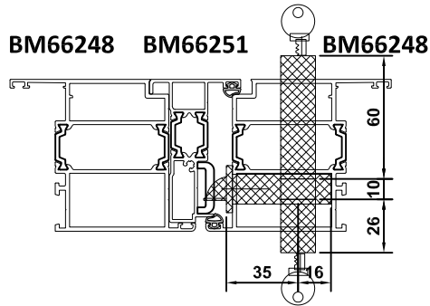
İÇE AÇILIR KAPI / INWARD OPENING DOOR
