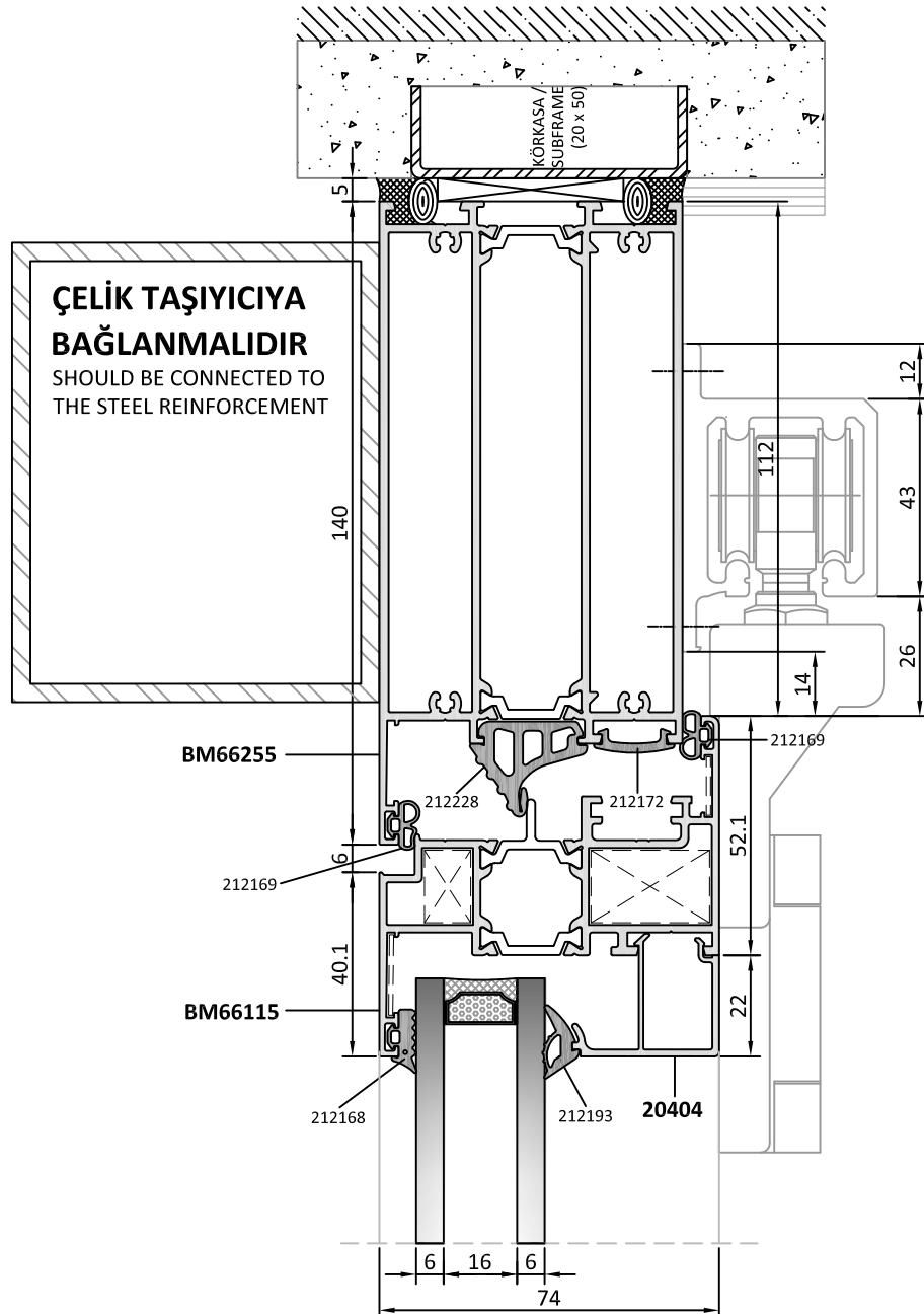
KATLANIR KAPI TİP 1 FOLDING DOOR TYPE 1
