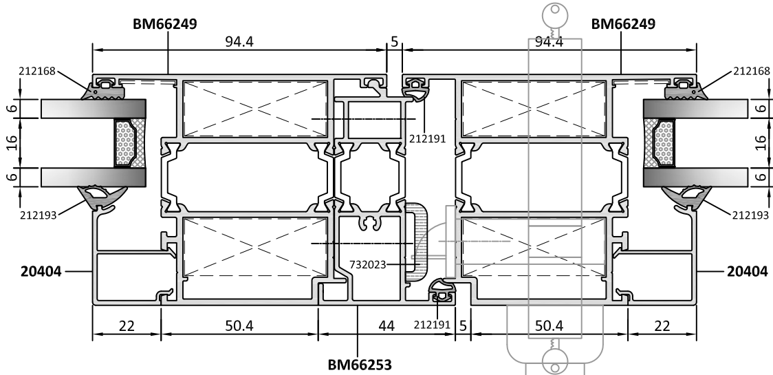
DIŞA AÇILIR KAPI OUTWARD OPENING DOOR
