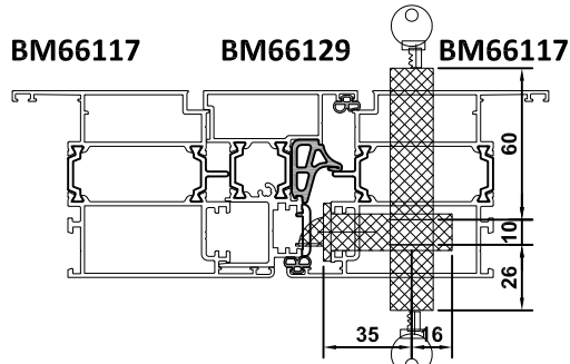
İÇE AÇILIR KAPI / INWARD OPENING DOOR
